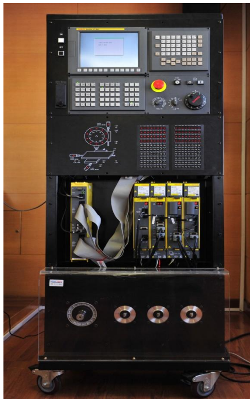
FANUC 0IMD 测试台
