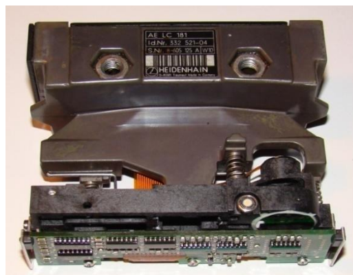
海德汉 AELS106 光栅头 增量式光栅尺 海德汉 AE LC181 绝对式光栅尺
